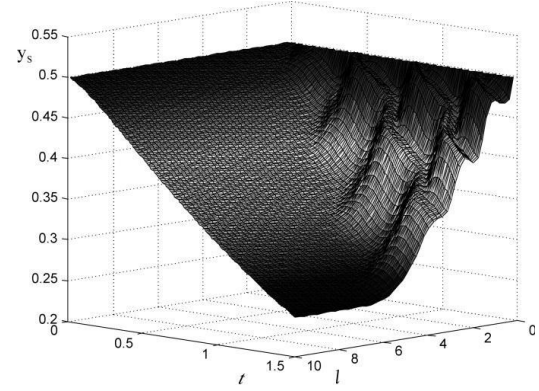
Şək.7. Hidrotəmizləmə reaktoru girişinə verilən xammal sürətinin periodik dəyişməsindən alınan qeyri-stasionar rejim.
