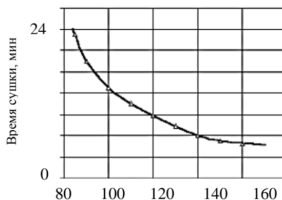
Рис. 2. Зависимость времени сушки от температуры сушки
