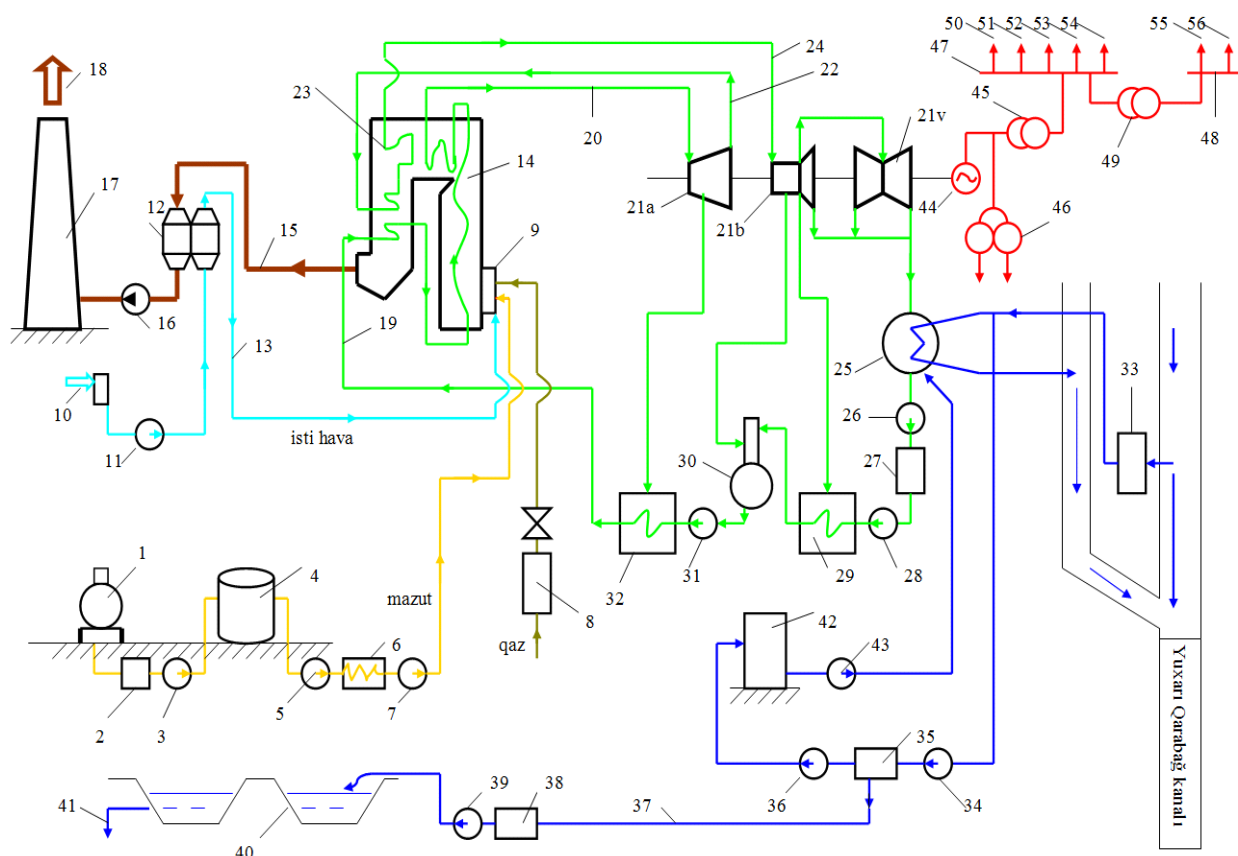
Şəkil 1. Azərbaycan İES-in texnoloji sxemi
